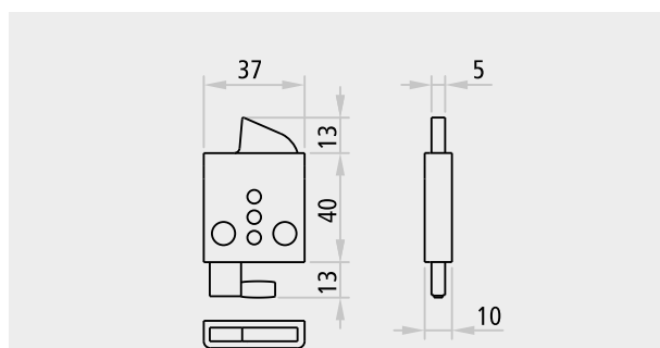
Horná re-západka zariadenie pre neaktívnu stranu Univer a REVER
