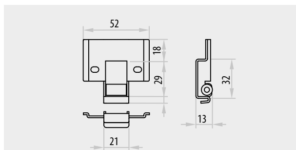
Horný box pre neaktívnu stranu PROGET a iné viacúčelové dvere
