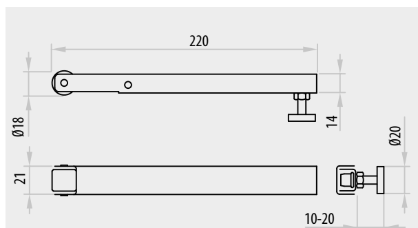
Nosné rameno pre krídla
