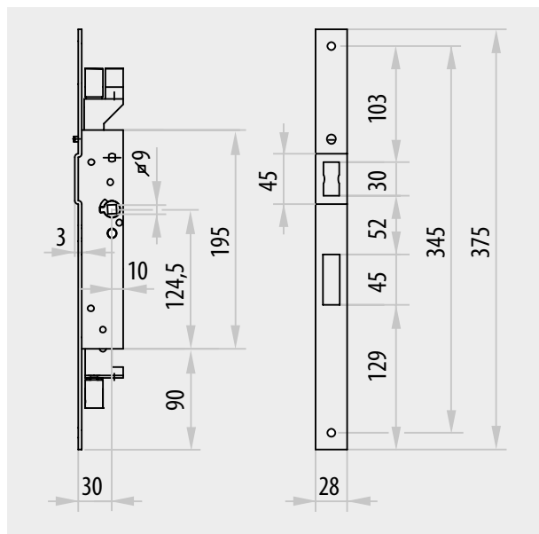
Poistka pre neaktívnu stranu
