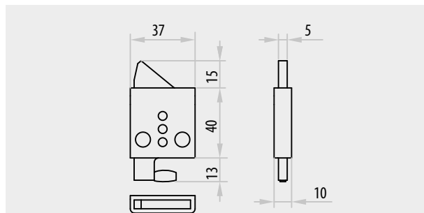
Horná re-západka zariadenie pre neaktívnu stranu PROGET a iných viacúčelových dverí
