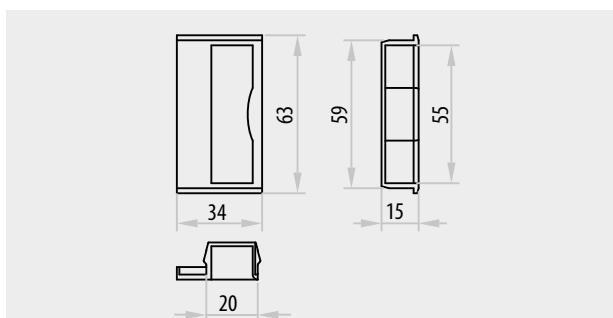
Doska vložka pre jednokrídlové dvere PROGET a iné viacúčelové dvere
