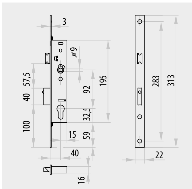
Zámok na jednokrídlové dvere alebo aktívne krídlo
