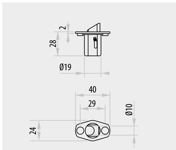
Horná re-západka pre neaktívnu stranu
